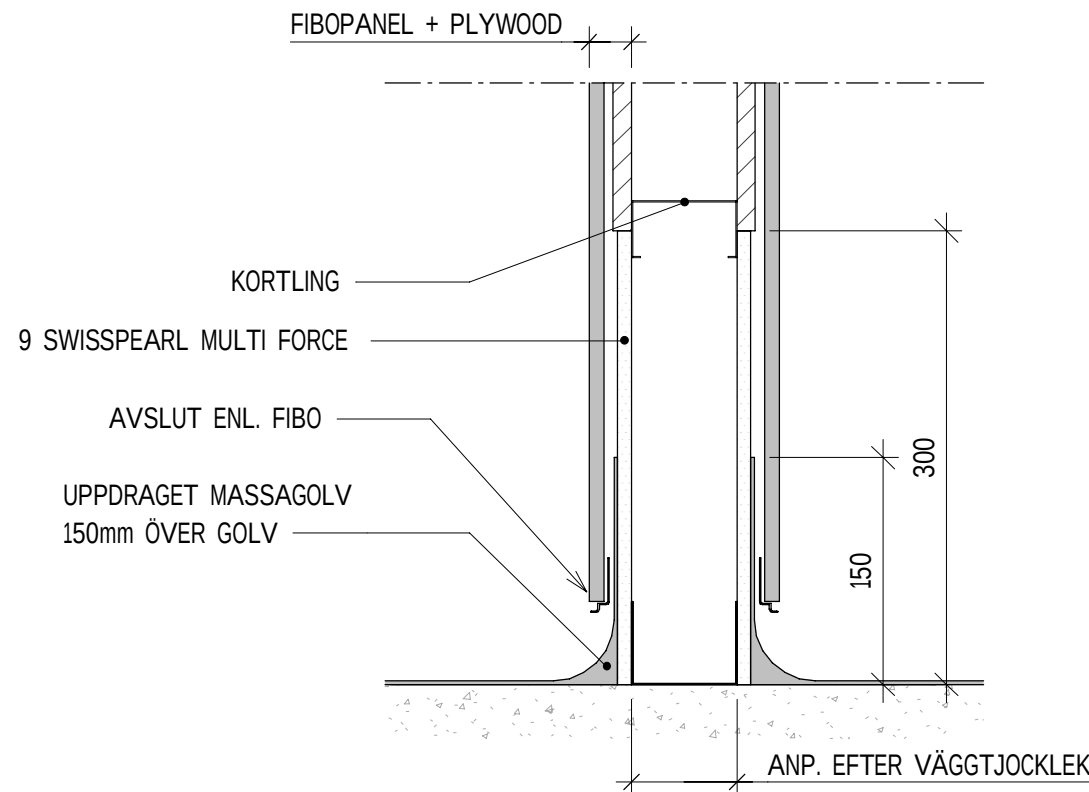
IVD10 - PRINCIPDETALJ MASSAGOLV MOT INNERVÄGG 1 : 5
