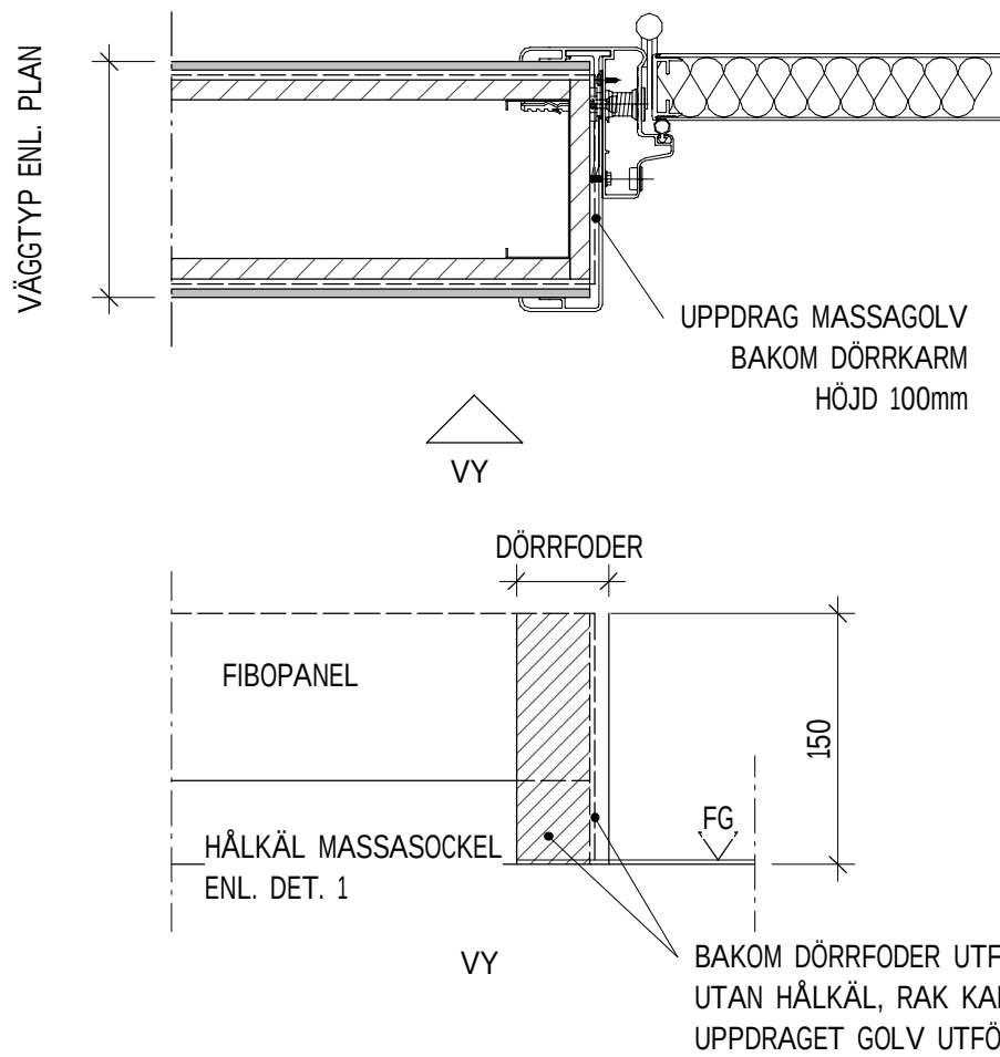
IVD03 - PRINCIPDETALJ INFÄSTNING DÖRRKARM AV GLASFIBER 1 : 5
