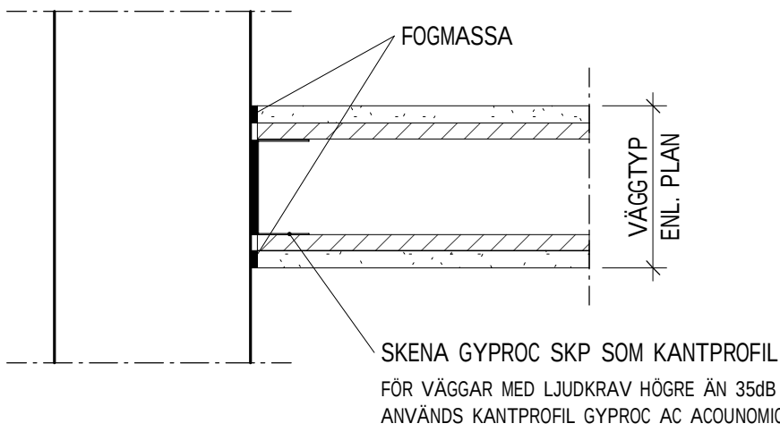
IVD01 - PRINCIPDETALJ MÖTE INNERVÄGG 1 : 5
