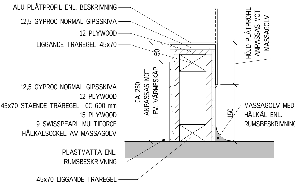
IVD14 - HÅLTAGNING VÄGG VÄRMESKÅP 1 : 5
