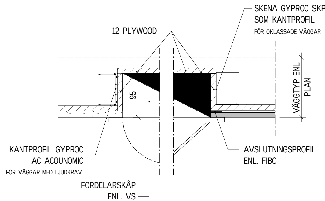
IVD06 - INKLÄDNAD FÖRDELARSKÅP 1 : 5
