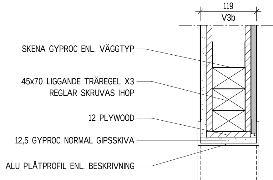
IVD13 - PRINCIPDETALJ TELESKOPANSLUTNING INNERVÄGG 1 : 5
