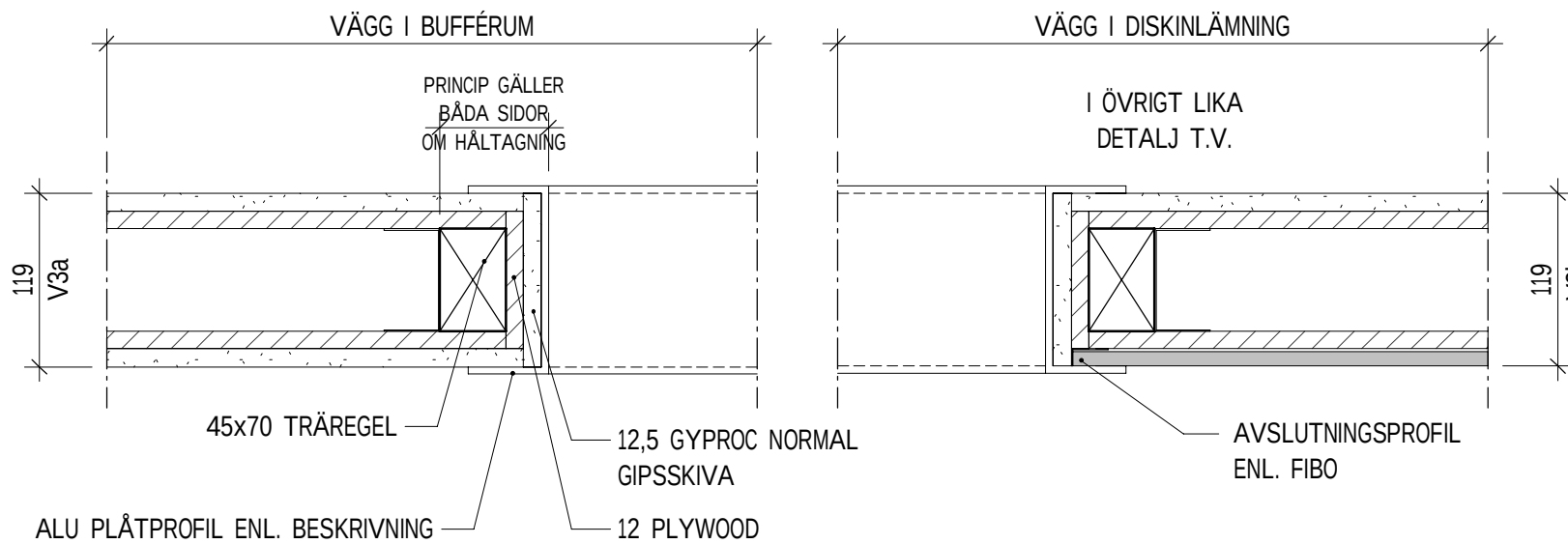
IVD07 - HÅLTAGNING VÄGG 1 : 5
